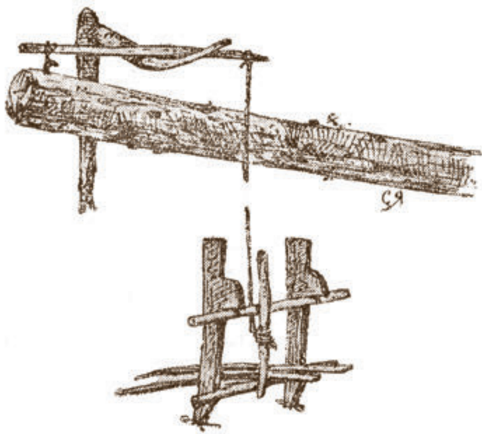
Механизм китайской ловушки на соболя, приводящий её в действие
