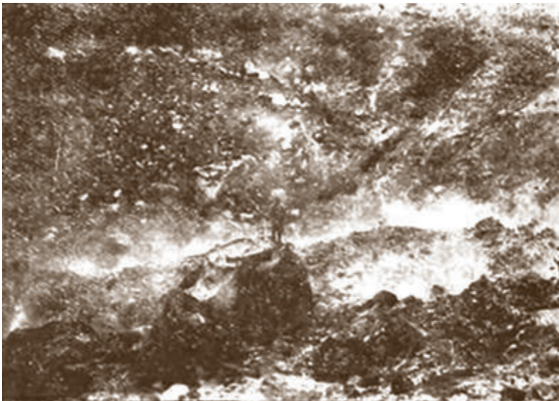
Дно воронки нового кратера Авачинского вулкана. Центральное поле мелких фумарол
